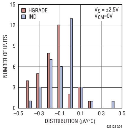
V_{OS} T_C (-40^\circ C \text{ to } 125^\circ C)
