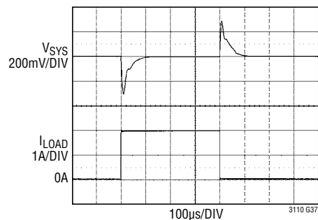
Load Step 0A to 2A
