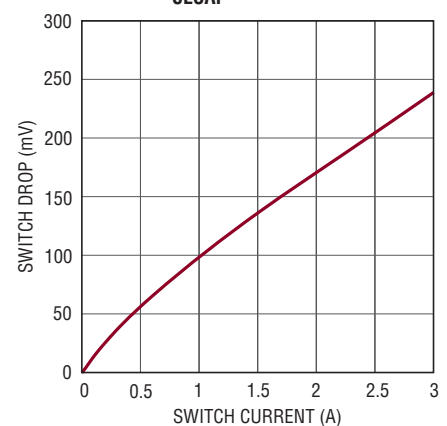
Switch V_{CESAT}
