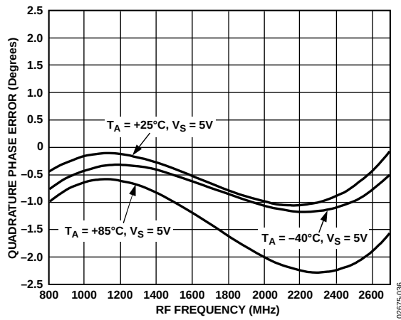
Figure 27. Quadrature Phase Error vs. F_{LO} , V_{GIN} = 0.7 V, V_S = 5 V
